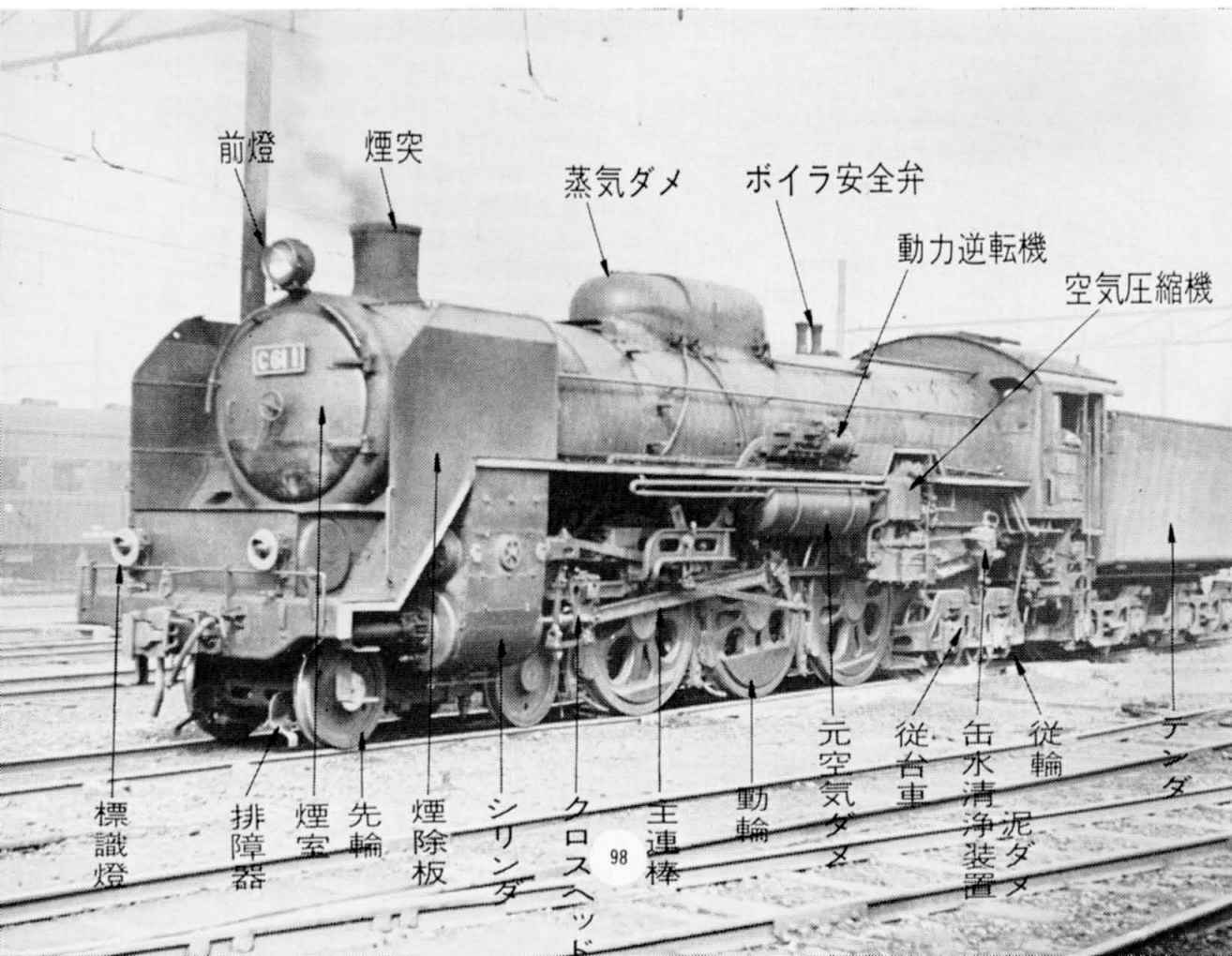
蒸気機関車の各部名称 (C61形)
